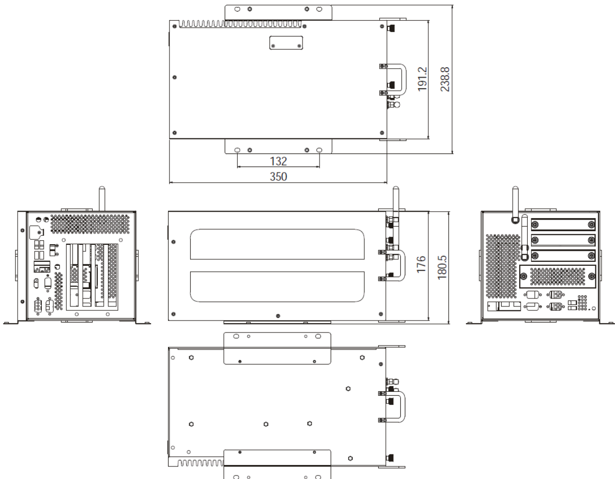
Вид спереди
